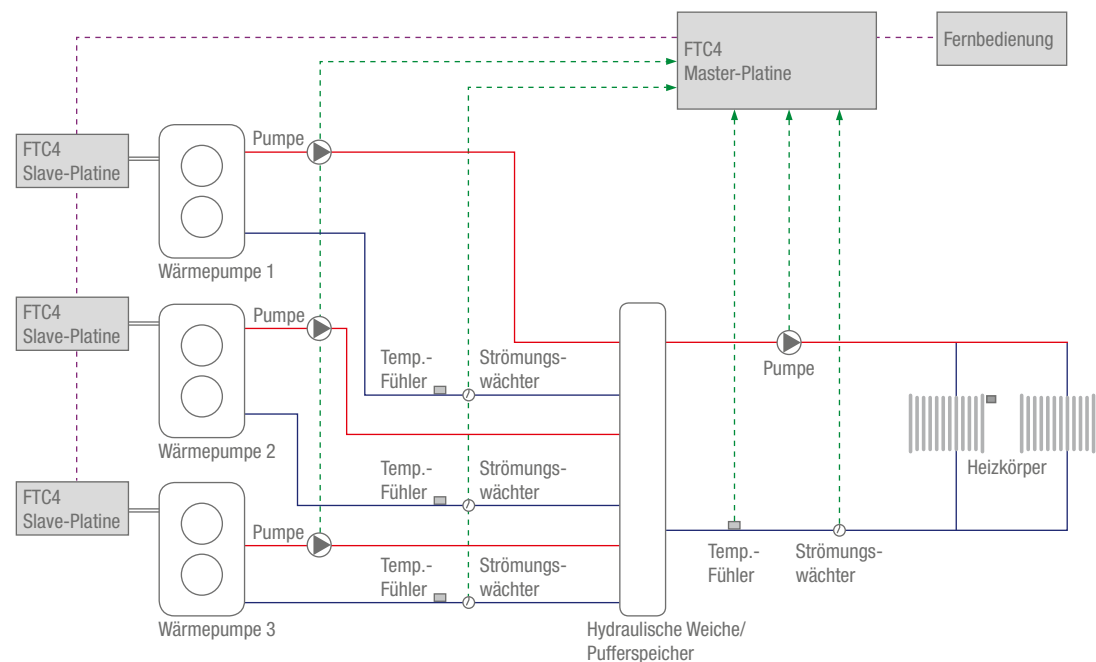
Schematische Darstellung einer 3er-Kaskade ohne Trinkwarmwasserbereitung
